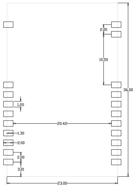
PCB LAYOUT(mm)
