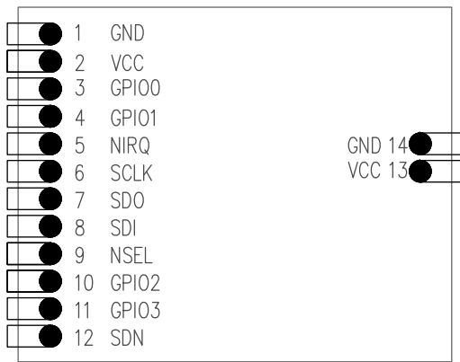
引脚说明
